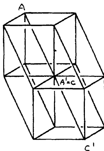
Figur 90 Schiefe Parallelprojektionen des Tesseractes
