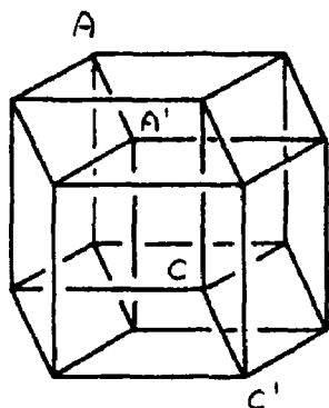
Figur 90 Schiefe Parallelprojektionen des Tesseractes
