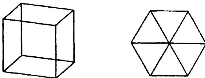
Figur 89 Orthogonale Parallelprojektionen des Würfels
